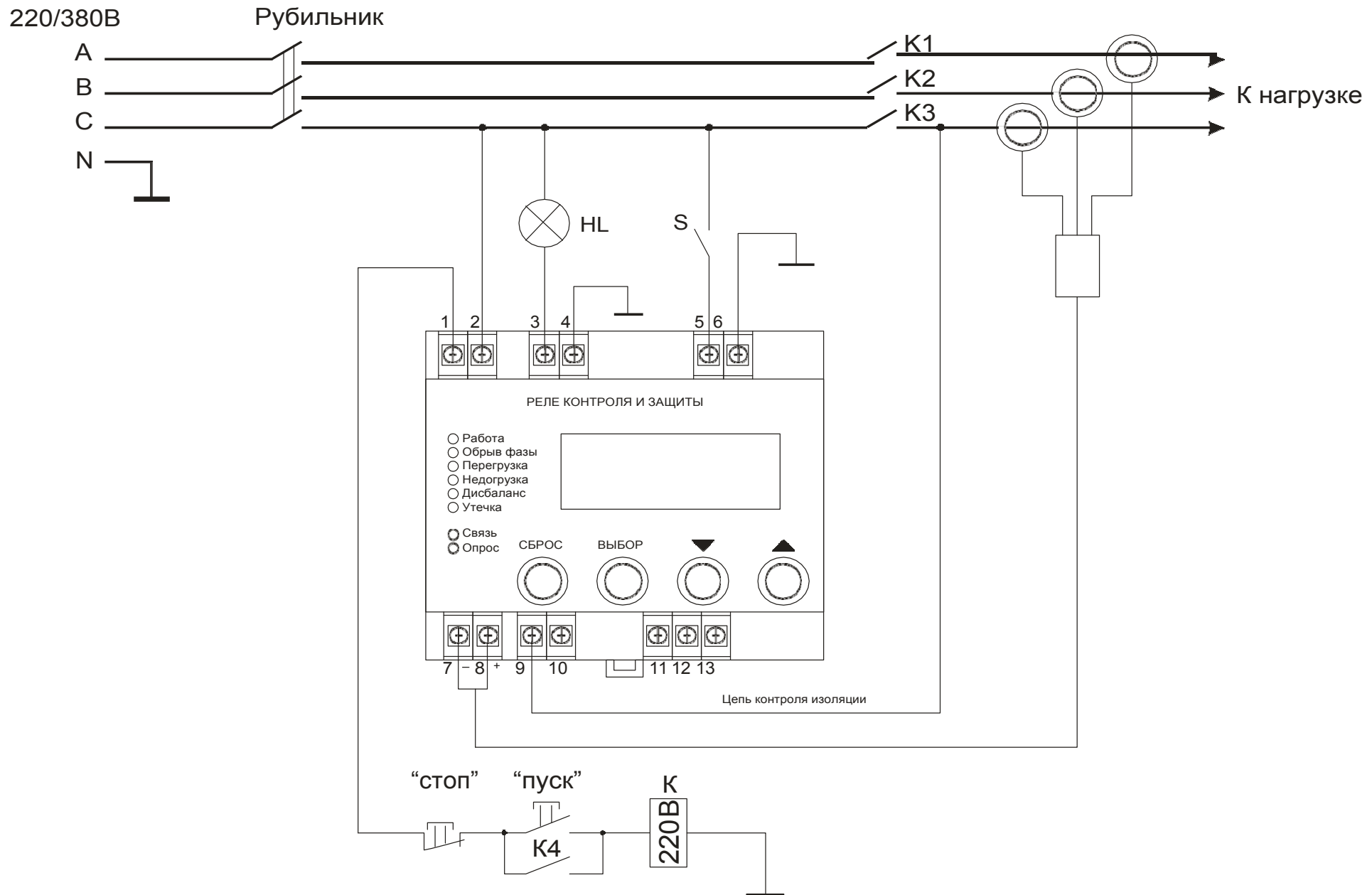
Рисунок 2 - схема включения реле РКЗМ-Д
